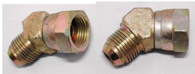
5番メス(東空・古河)x4番オス(オカダ) ブロック45° エルボ
