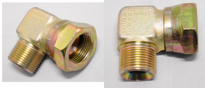
4番メス(オカダ)×5番オス(東空・古河) ブロック90° エルボ
