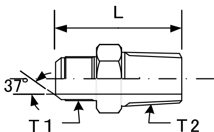
1013ユニファイ (異径PT大)
