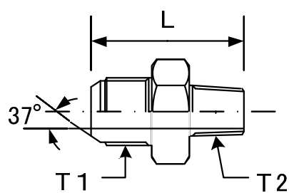
1013ユニファイ (異径PT小)
