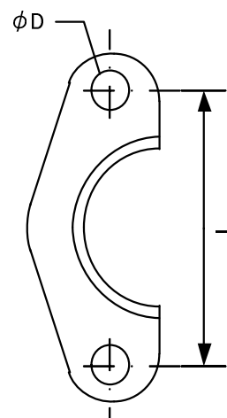
割フランジ (6000PSI用スプリットフランジ)
