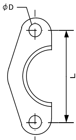
割フランジ (3000PSI用スプリットフランジ)
