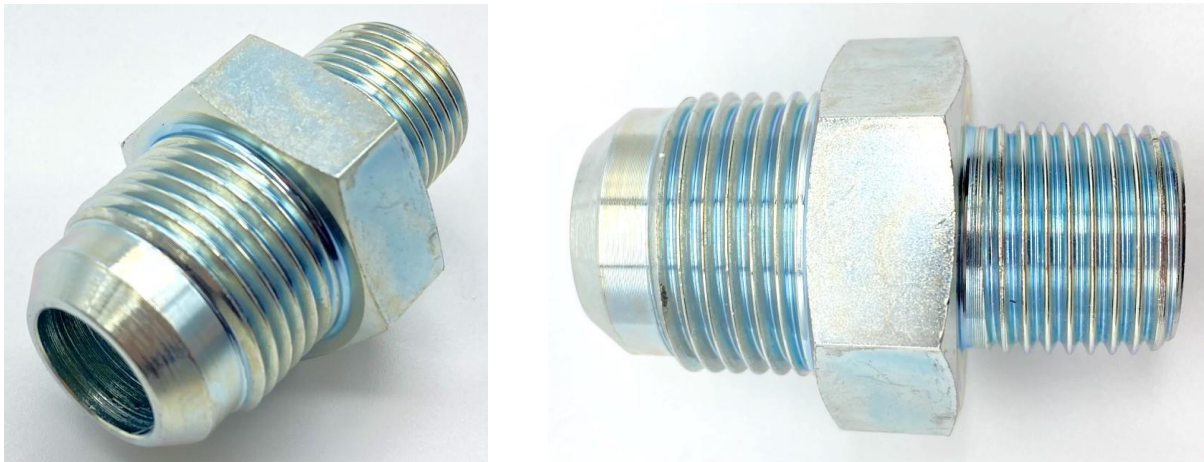
③ 1013ユニファイ (異径PT小)
